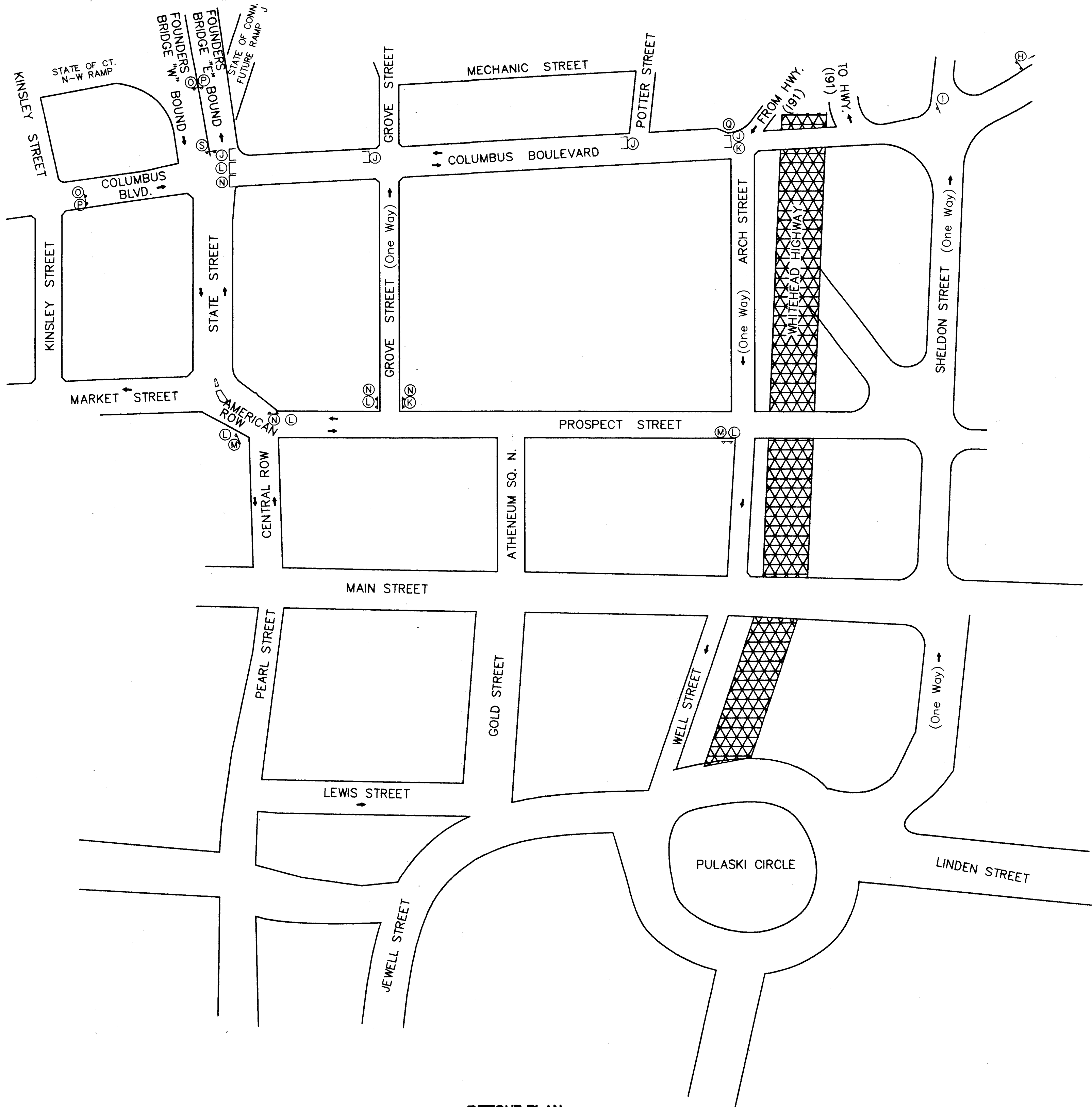
DETOUR PLAN SCALE 1:2 000
