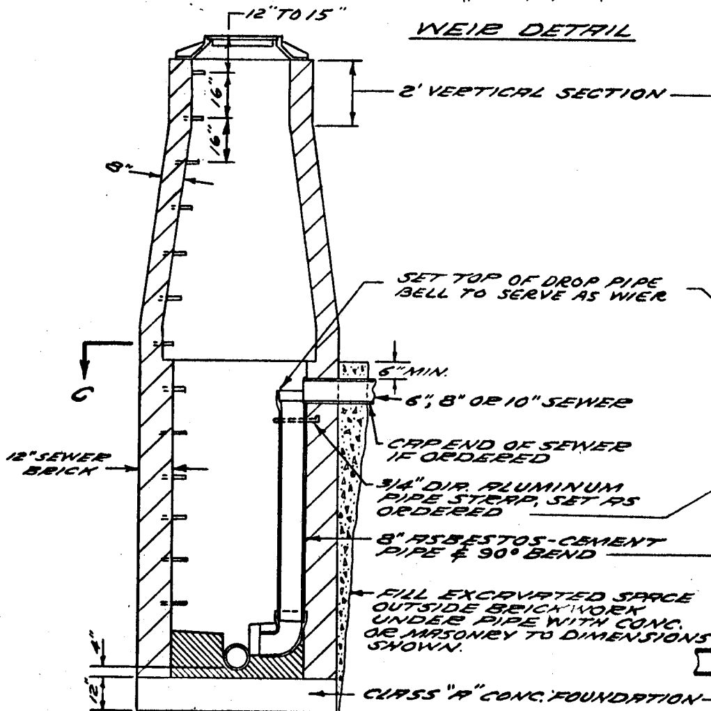
SECTION A-A
