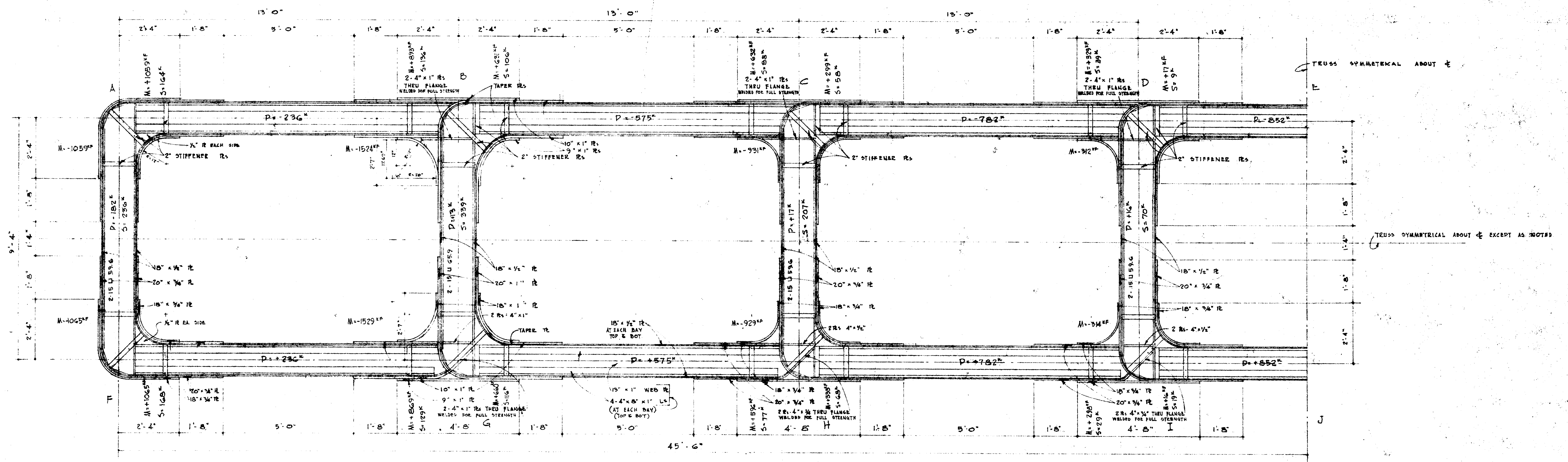
VIERENDEEL TRUSS 'A' SCALE: 1/8"=1'-0"
