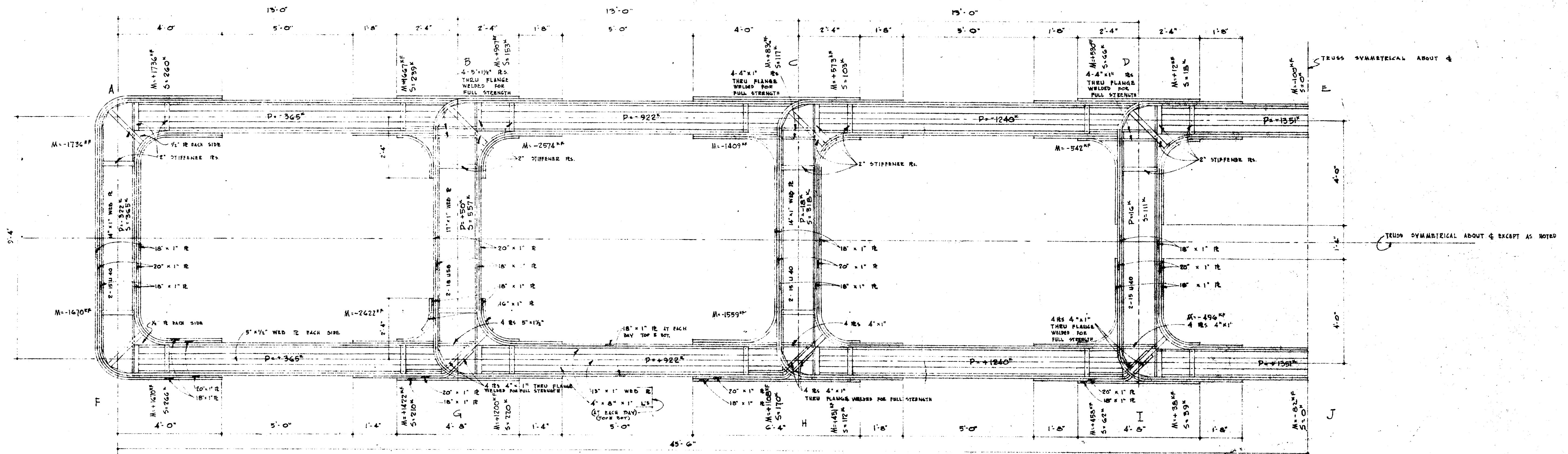
VIERENDEEL TRUSSES 'B' & 'C' SCALE: 1/8"=1'-0"
