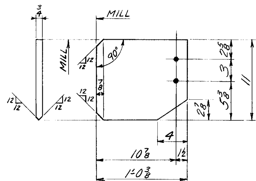
12- PLATES MK. A1-10; A2-10 (6EA.)
