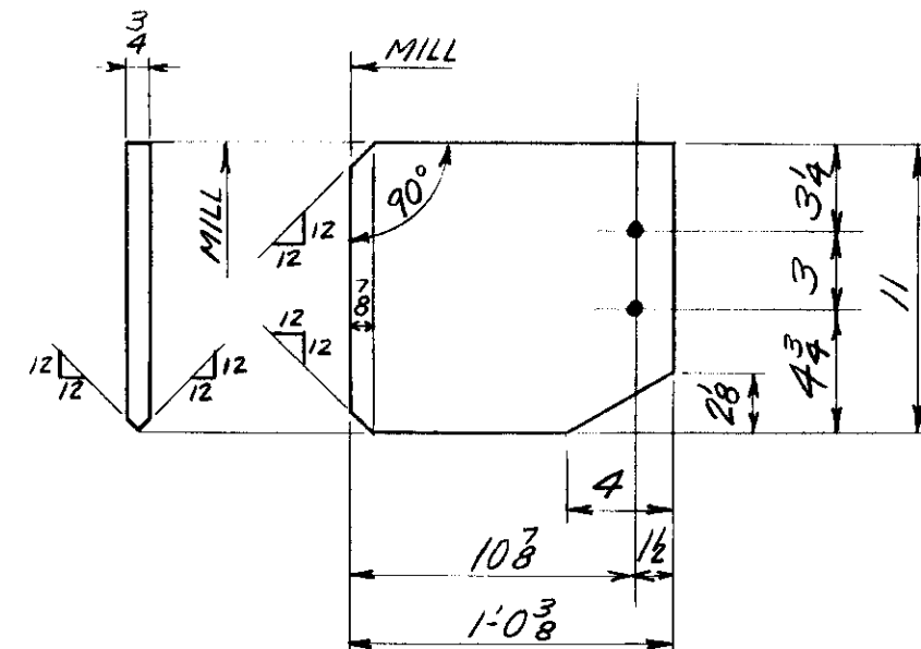
6-PLATES MK. A1-11; A2-11 (3EA.)
