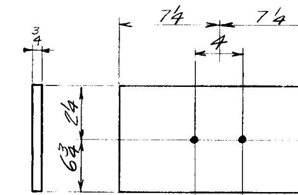
4-PLATES MK. A1-13; A2-13 (2EA)
