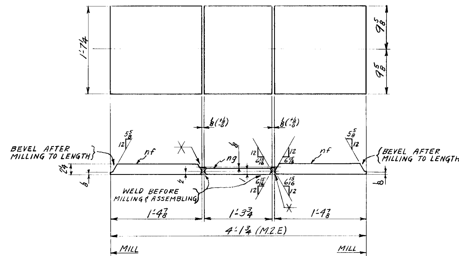
8 - PLATES MK. nf 4 - PLATES MK. ng
