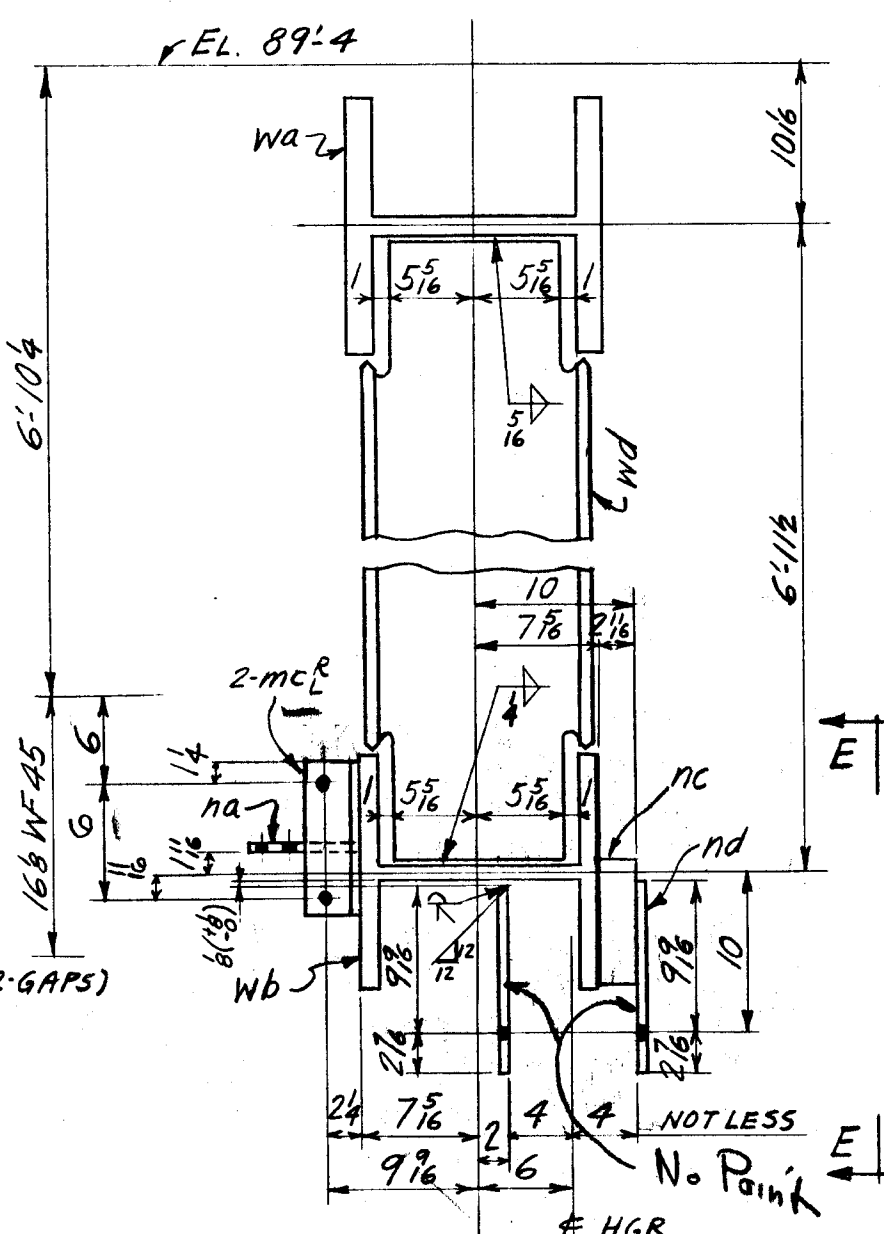
SECTION D-D
