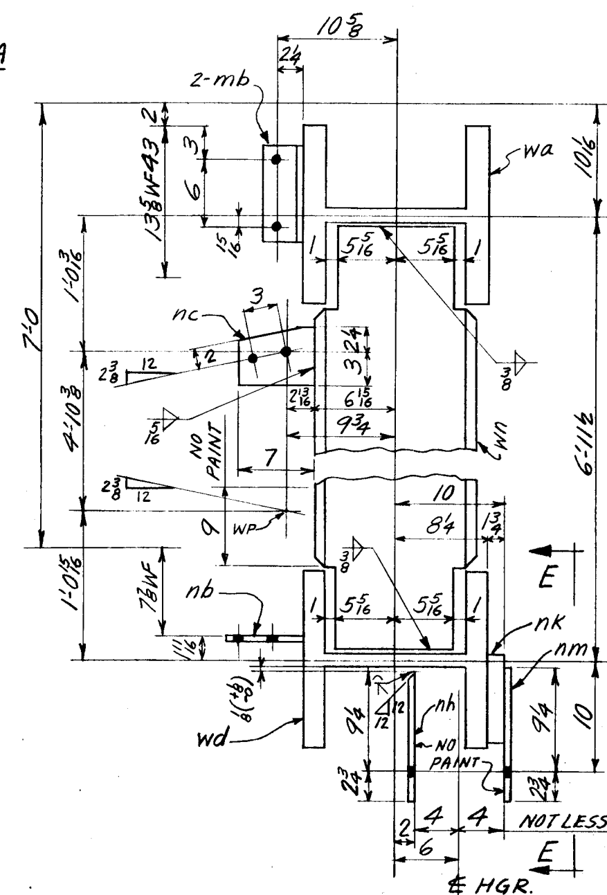
SECTION A-A
