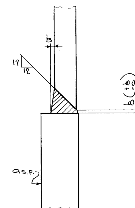
SECTION 15-15
