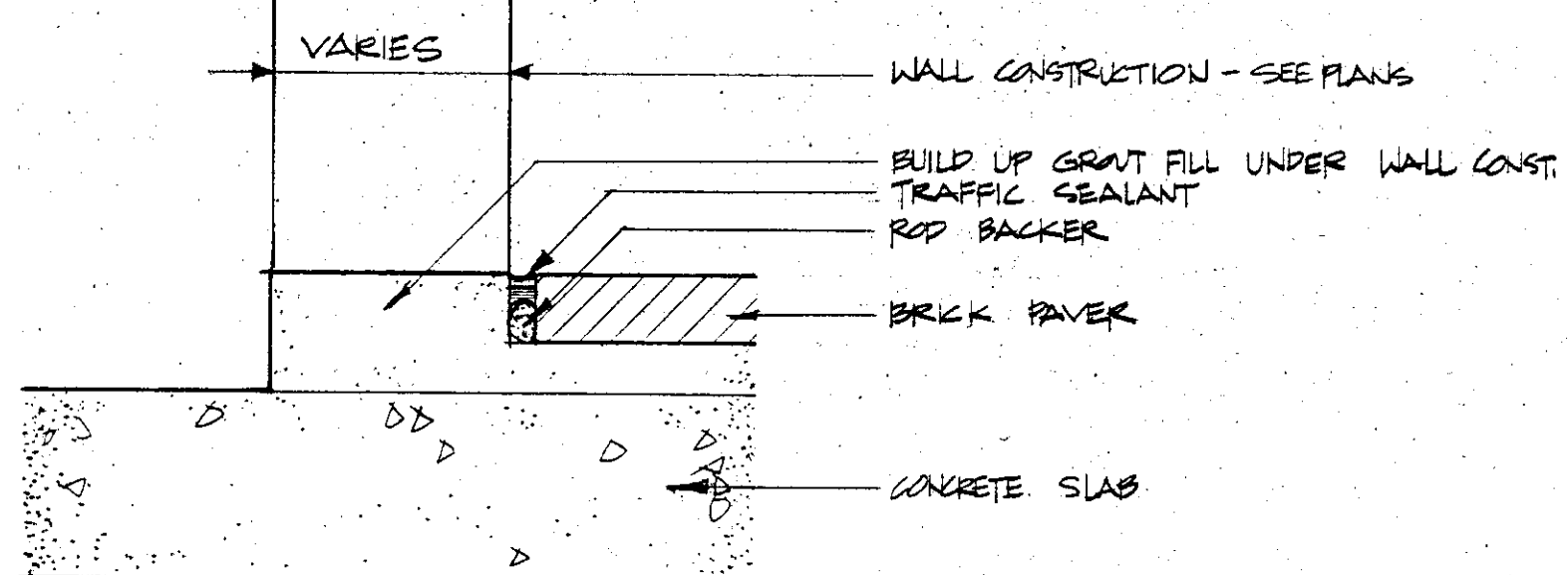
2 DETAIL SCALE: 3" = 1'-0"
