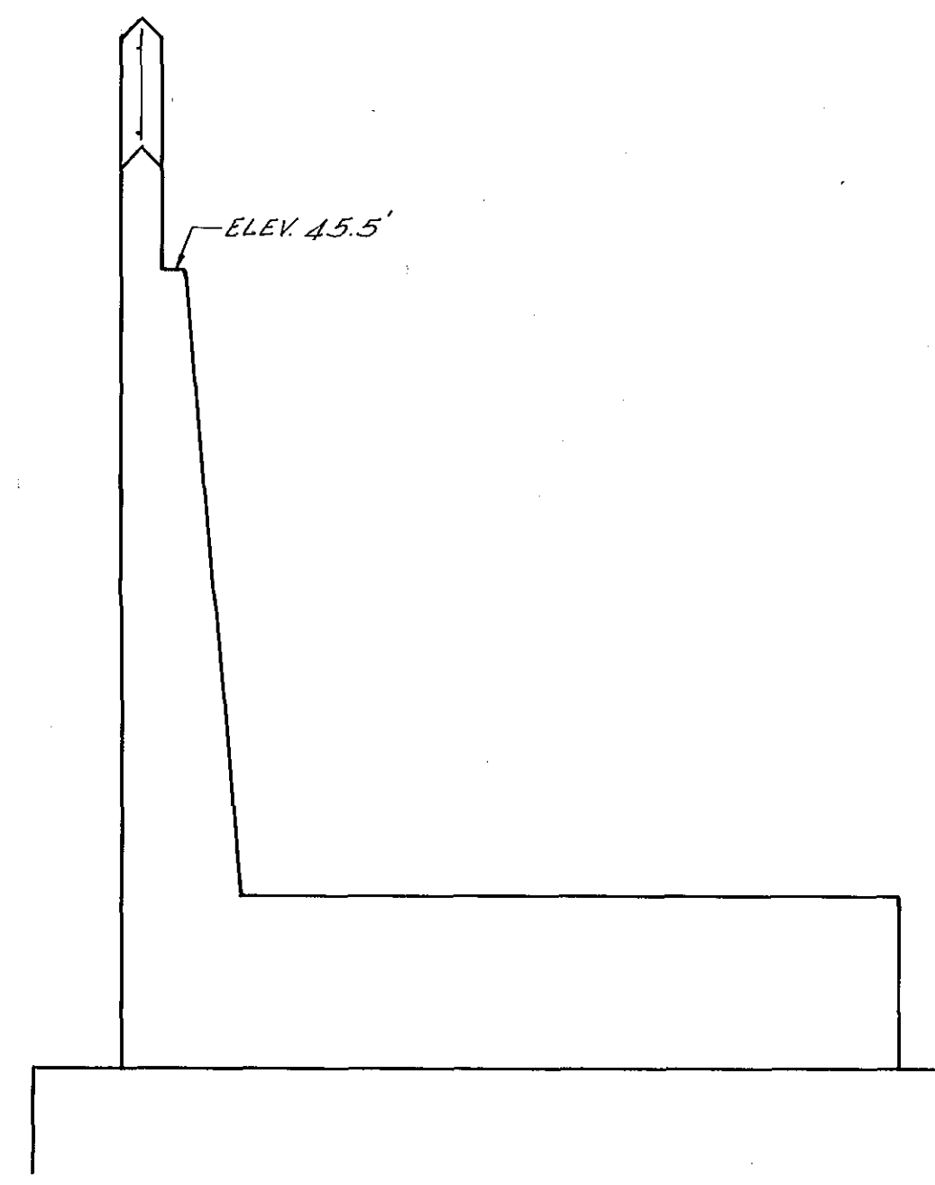
SECTION D-D
