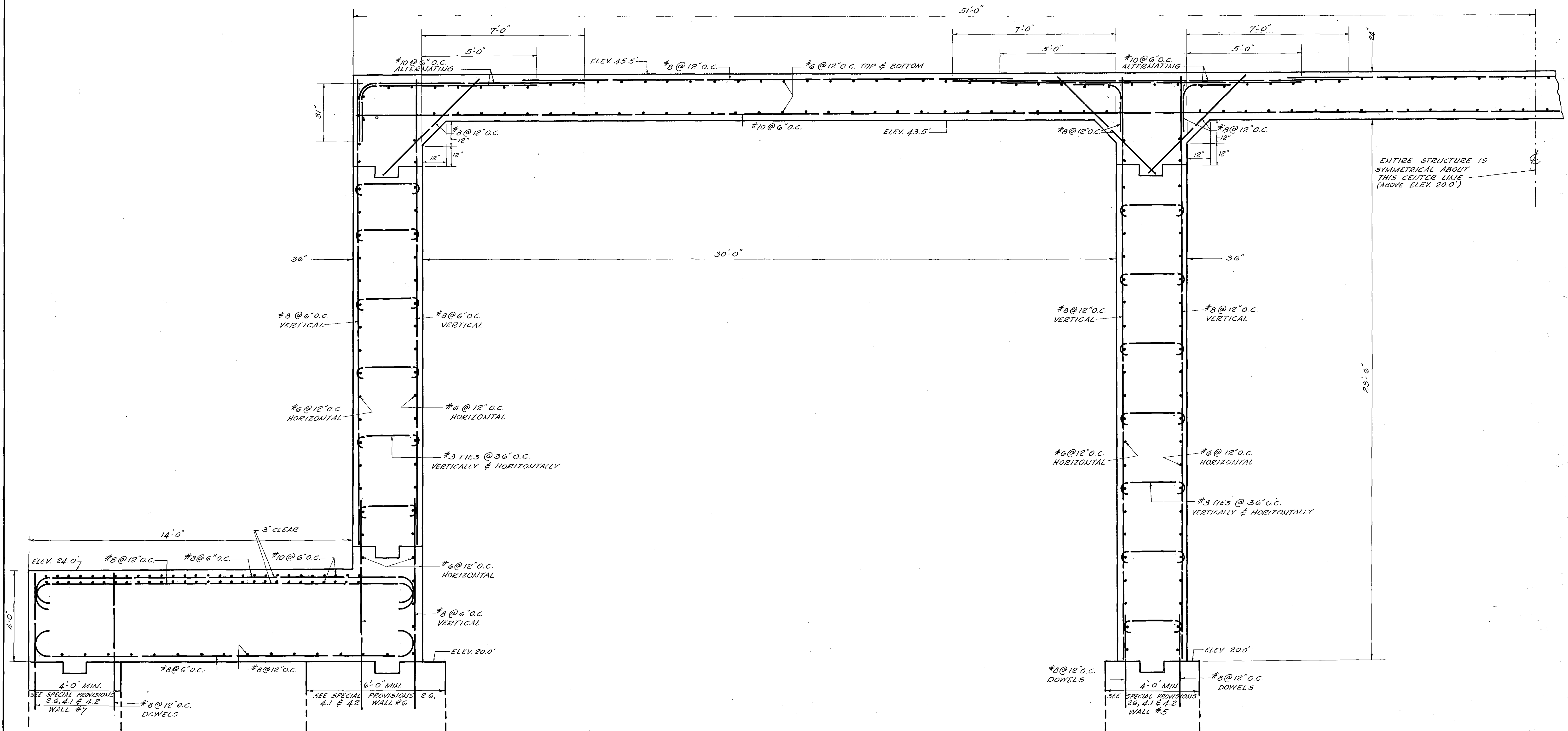
SECTION A-A
